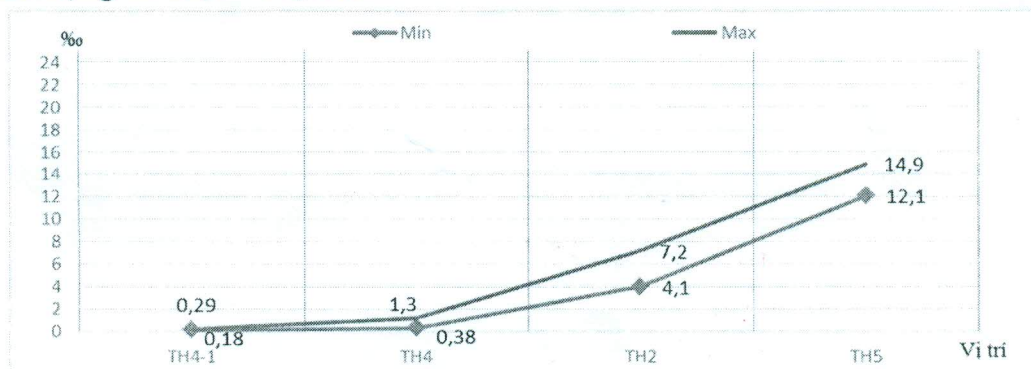
Hình 1: Biểu đồ độ mặn trên sông Thạch Hãn
